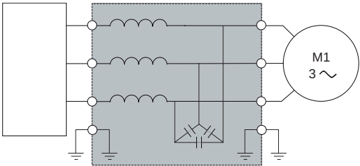
Синусный фильтр
